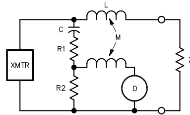
Carey-Foster (Twin-Lamp, Monomatch Mickey-Match) (D)
